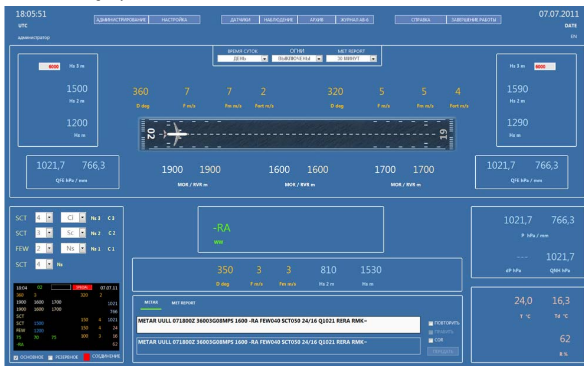
Рисунок 2. Главное окно станции АМС «ЛОМО-МЕТЕО-01»
